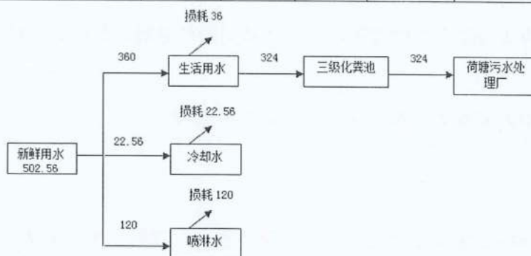
图 3.5 项目水平衡图(单位: t/a)
