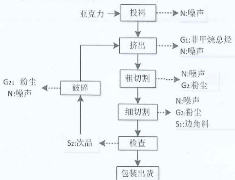
图 3.6 本项目生产工艺流程图
