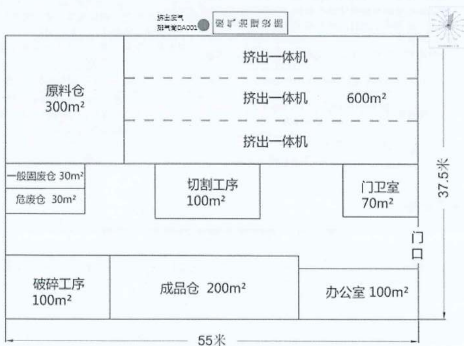
附图 3.3 项目厂区总平面布置图
