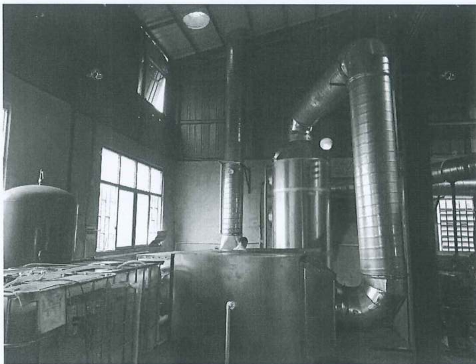
图 4.2 熔铝、脱模废气治理设施图
