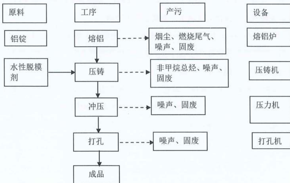
图 3.6 项目生产工艺流程及产污环节示意图
