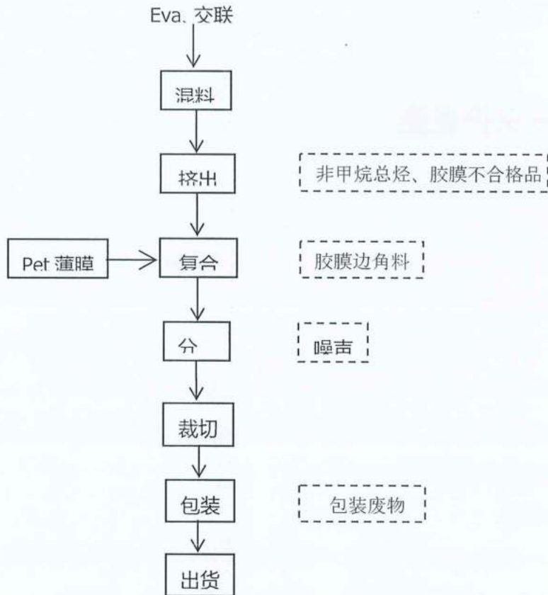
图 3.6 生产工艺流程及产污环节示意图
