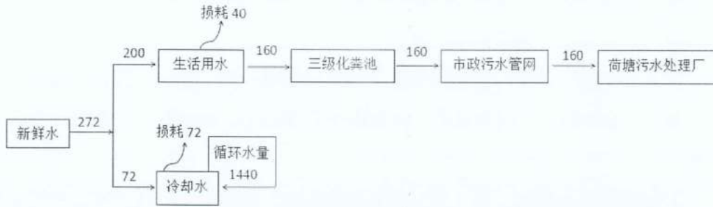
图 3.5 项目水平衡图(单位: m^3/a )
