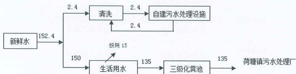
图3.5 项目平衡图 (单位: t/a)
