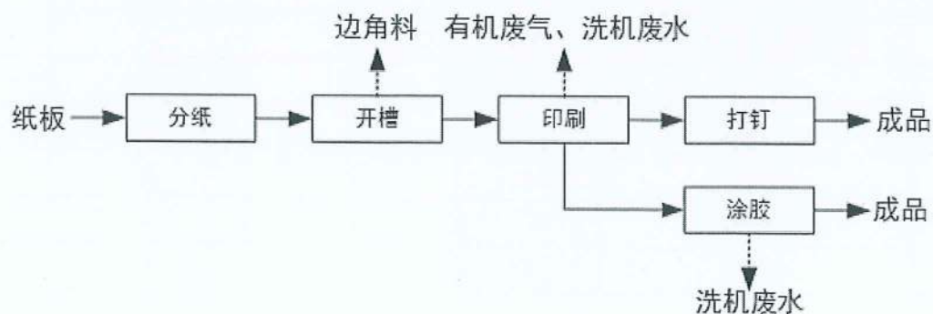
图 3.6 项目生产工艺流程图
