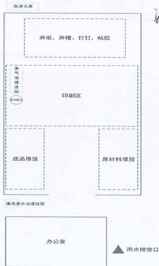
图 3.4 项目车间平面布置图
