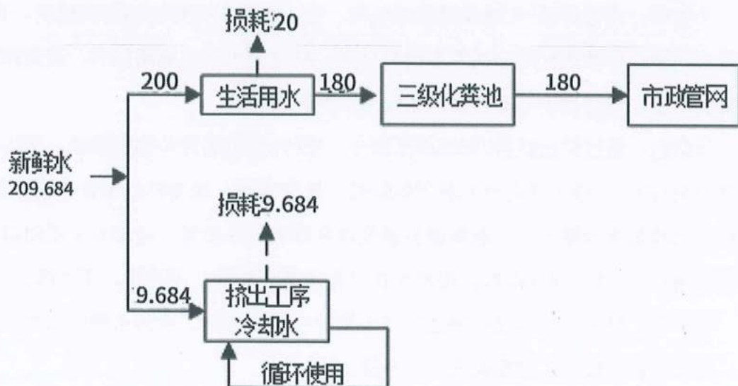
图3-6项目平衡图 (单位: t/a)
