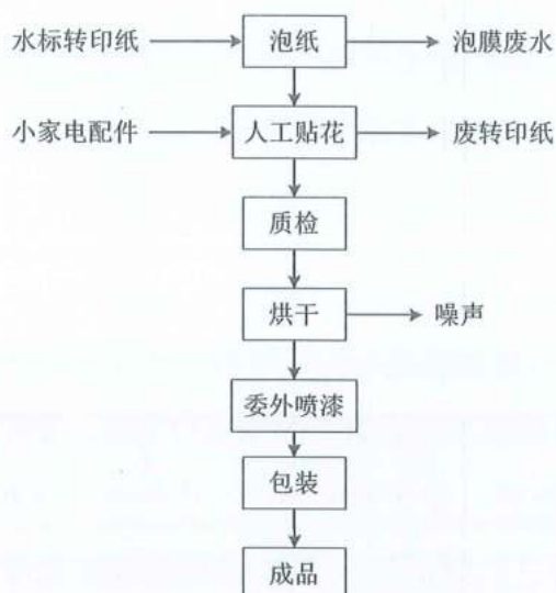
图 3-8项目营运期生产工艺流程及产污环节图
