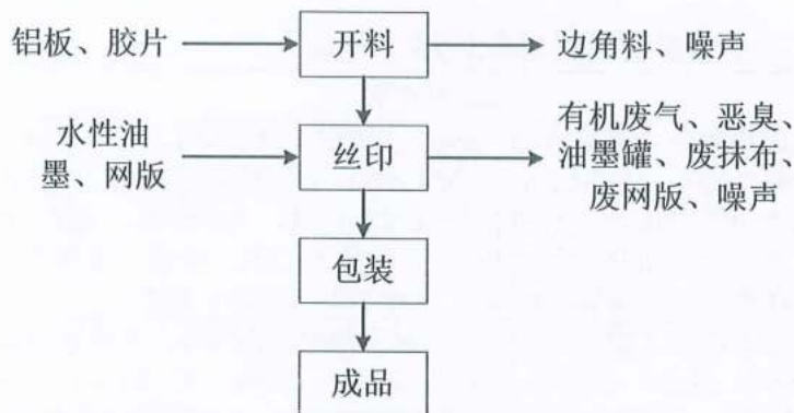
图 3-7 项目营运期生产工艺流程及产污环节图
